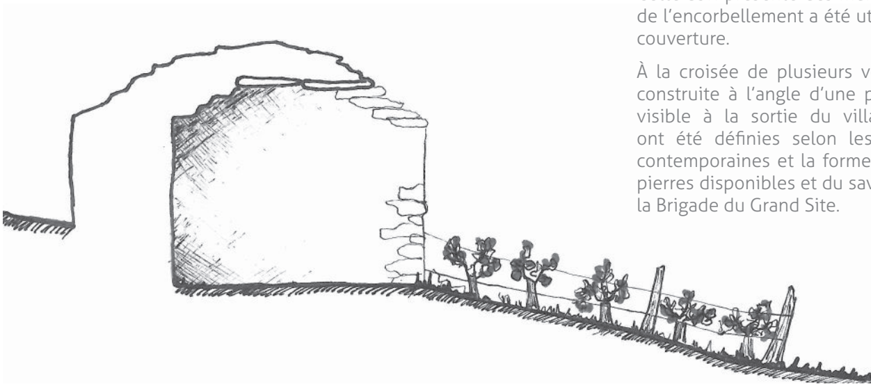
← Coupe AA' de la cadole
